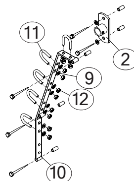
Avslutning mot vegg, for rørfront
