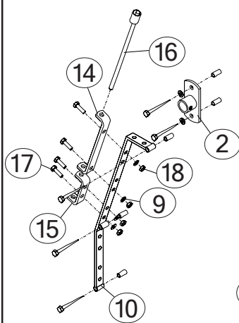
Avslutning mot vegg, for port
